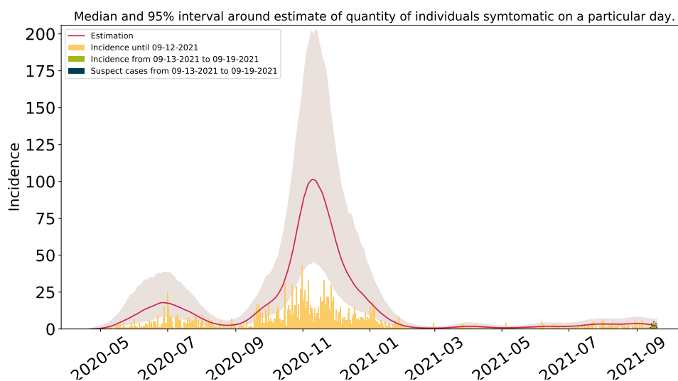
Figura 40: Estimación del número de enfermos sintomáticos en Cananea. Estimación sustentada en la proporción de infecciones sintomáticas de acuerdo a las distribuciones de covidestim ajustadas a los datos de México.
