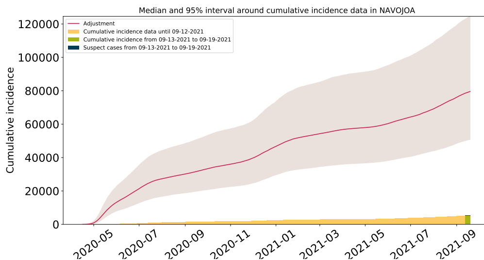
Figura 87: Ajuste y estimación de casos positivos acumulados de COVID-19 por inicio de síntomas en Navojoa.
