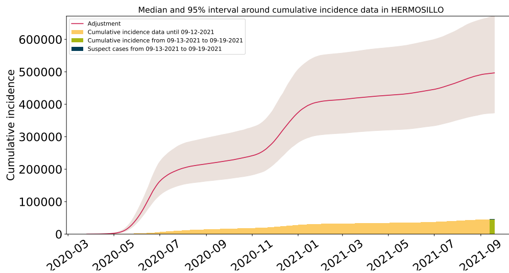
Figura 66: Ajuste y estimación de casos positivos acumulados de COVID-19 por inicio de síntomas en Hermosillo.
