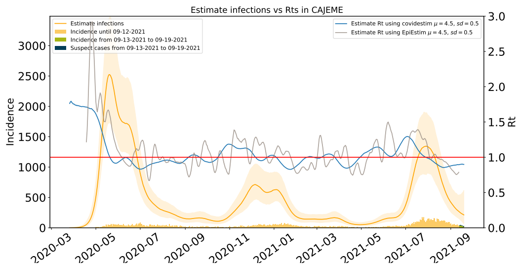
Figura 35: Comparación de las estimaciones de R_t con covidestim y EpiEstim. La figura muestra también el total de infecciones estimadas en Cajeme para efectos comparativos. R_t con covidestim está calculado con base en las infecciones totales estimadas y se calcula hasta 7 días antes de la fecha de actualización de la base de datos. R_t con EpiEstim usa las infecciones reportadas y se calcula hasta 14 días antes de la fecha de actualización de la base de datos. Ambos métodos rinden tendencias similares, en lo general, pero no son iguales.
