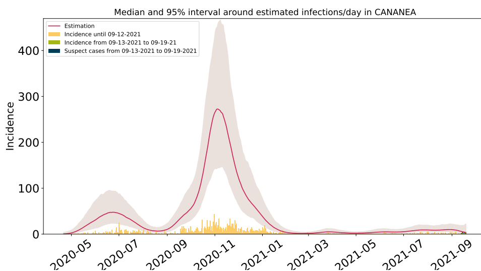
Figura 41: Estimación de infecciones diarias por COVID-19 en Cananea. Estimación sustentada en la proporción de infecciones totales de acuerdo a las distribuciones de covidestim ajustadas a los datos de México.
