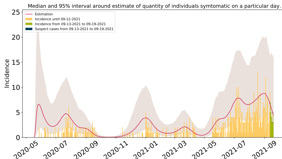
Figura 19: Estimación del número de enfermos sintomáticos en Benito Juárez. Estimación sustentada en la proporción de infecciones sintomáticas de acuerdo a las distribuciones de covidestim ajustadas a los datos de México.
