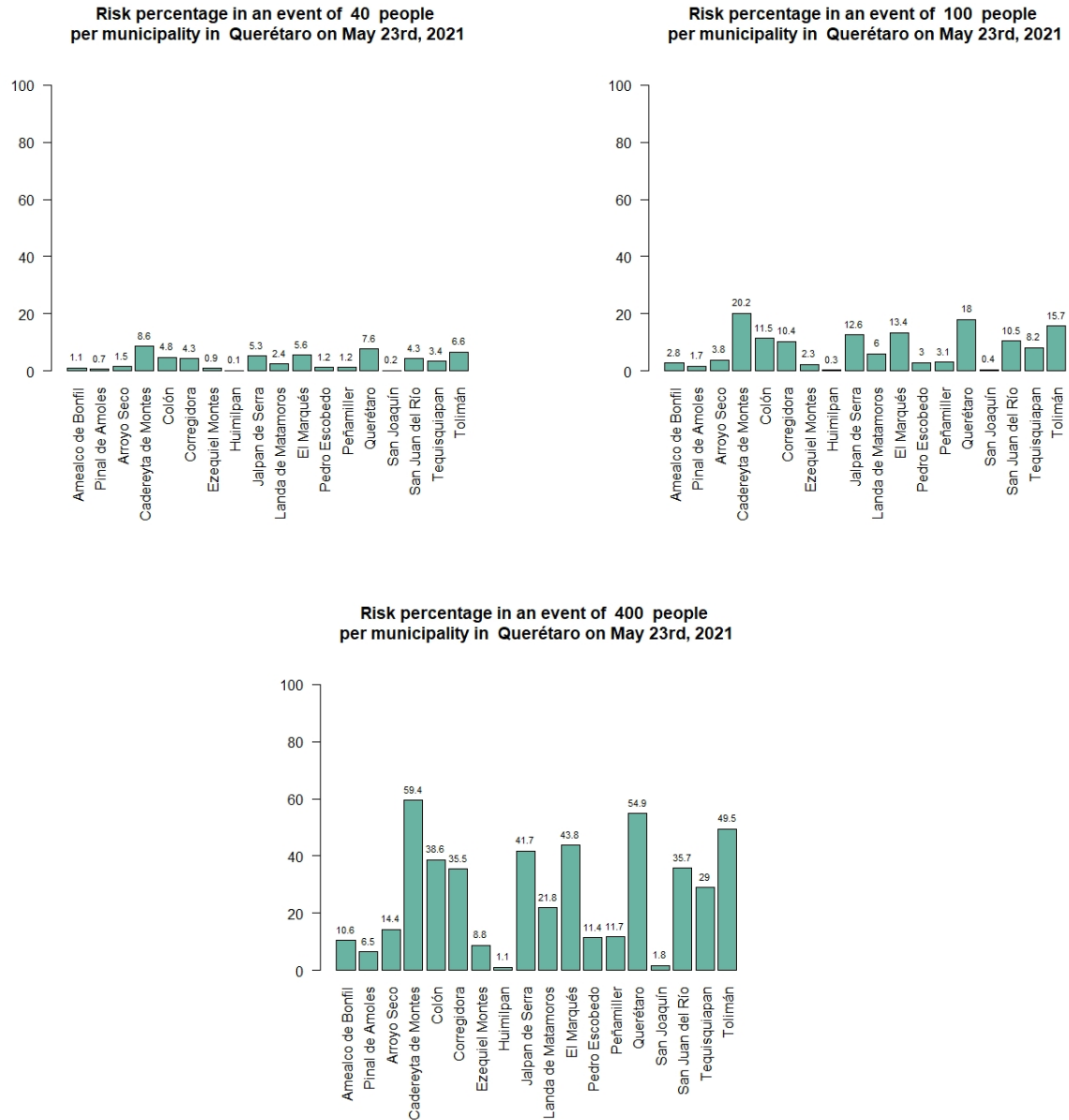
Cuadro 6: Porcentajes de riesgo de contagio por COVID-19 para cada municipio del estado de Querétaro, en eventos con aforo de 40, 100 y 400 personas al 23 de mayo de 2021. Estimaciones calculadas con datos de [2] actualizados el 30 de mayo y recortados hasta el 23 de mayo.
