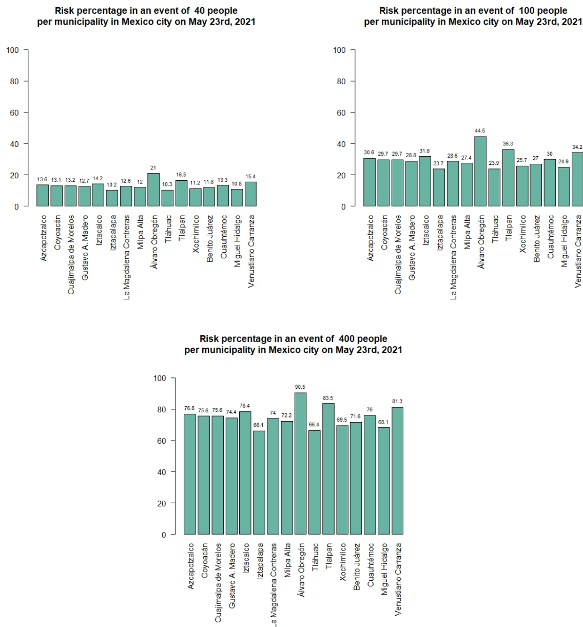
Cuadro 4: Porcentajes de riesgo de contagio por COVID-19 para cada alcaldía de CDMX, en eventos con aforo de 40, 100 y 400 personas al 23 de mayo de 2021. Estimaciones calculadas con datos de [2] actualizados el 30 de mayo y recortados hasta el 23 de mayo.
