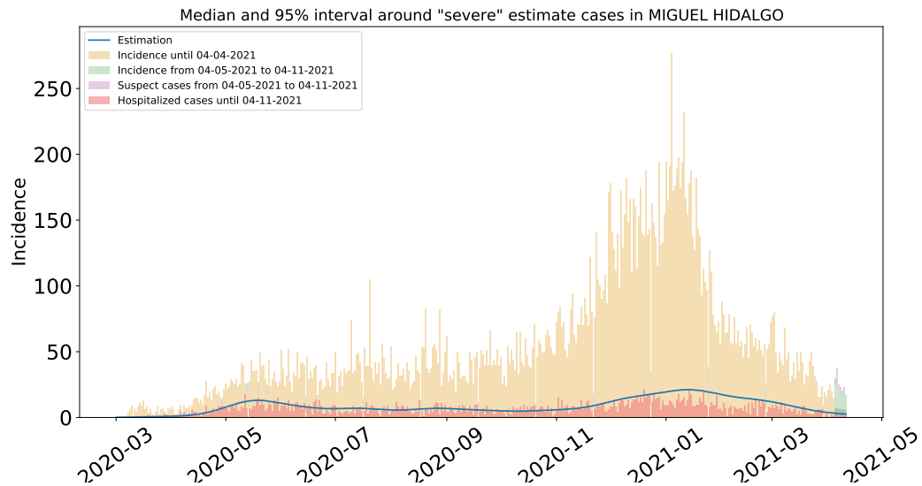
Figura 69: Estimación de casos severos de COVID-19 en la alcaldía de Miguel Hidalgo comparada con los casos hospitalizados reportados.
