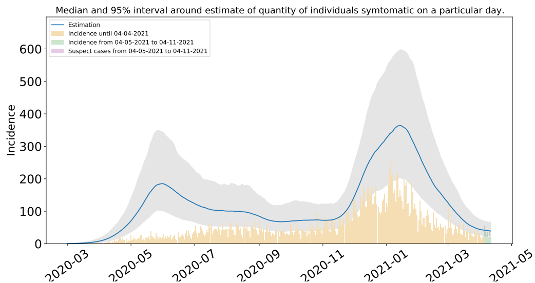
Figura 64: Estimación del número de enfermos sintomáticos en Magdalena Contreras. Estimación sustentada en la proporción de infecciones sintomáticas de acuerdo a las distribuciones de covidestim (Cuadro 4 del Apéndice metodológico).
