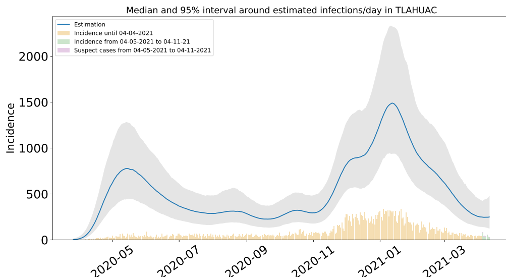
Figura 83: Estimación de infecciones diarias por COVID-19 en Tlaxiaco. Estimación sustentada en la proporción de infecciones totales de acuerdo a las distribuciones de covidestim (Cuadro 4 del Apéndice metodológico).
