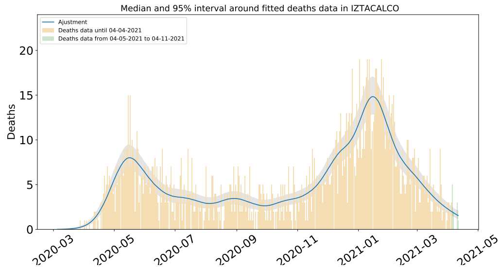
Figura 50: Ajuste y estimación de defunciones por COVID-19 para la alcaldía de Iztacalco.
