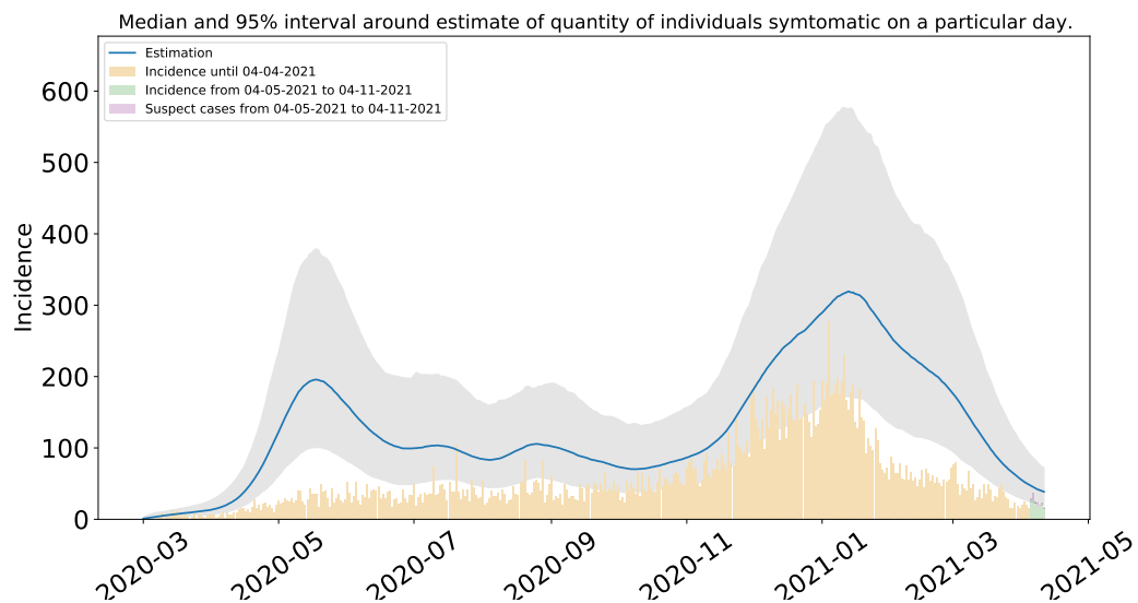
Figura 70: Estimación del número de enfermos sintomáticos en Miguel Hidalgo. Estimación sustentada en la proporción de infecciones sintomáticas de acuerdo a las distribuciones de covidestim (Cuadro 4 del Apéndice metodológico).
