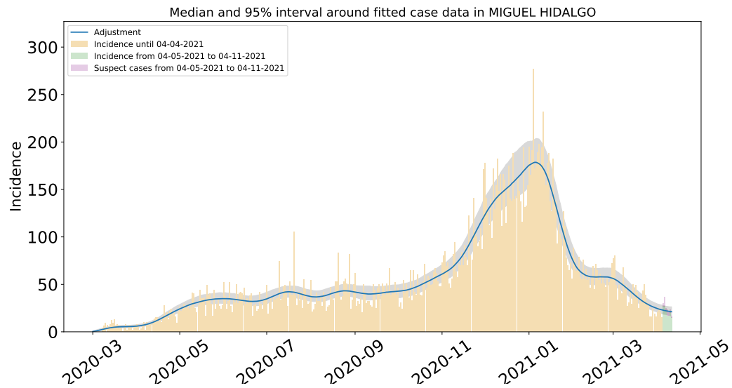
Figura 67: Ajuste de casos positivos (incidencia) por inicio de síntomas de COVID-19 en Miguel Hidalgo.
