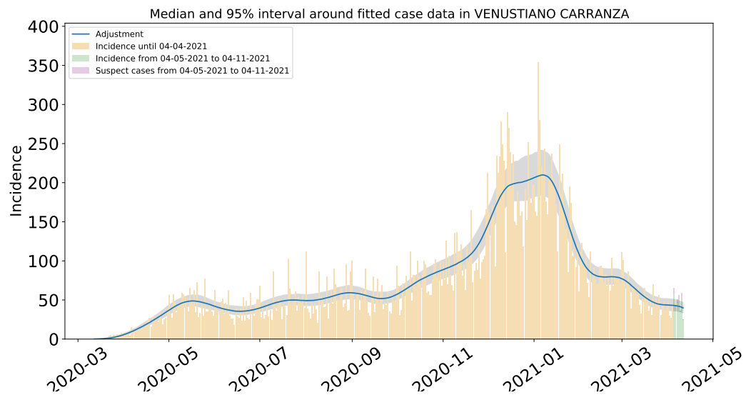
Figura 97: Ajuste de casos positivos (incidencia) por inicio de síntomas de COVID-19 en Venustiano Carranza.
