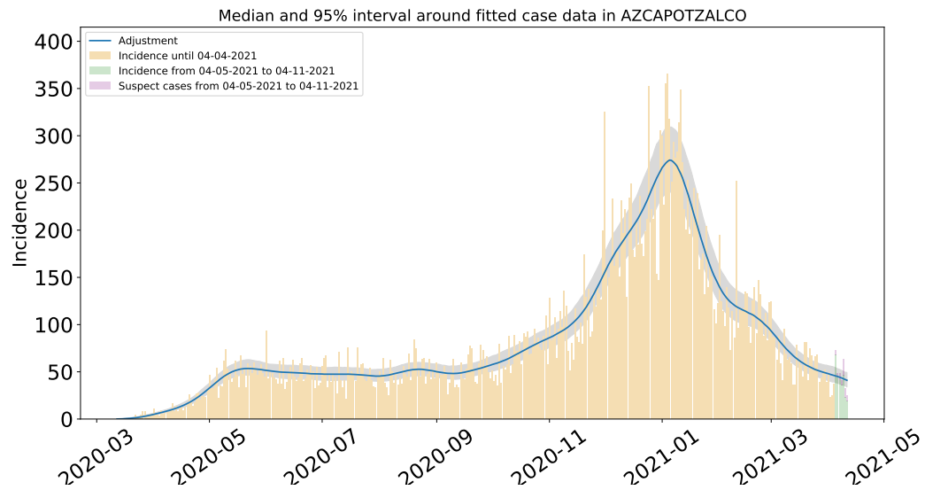
Figura 13: Ajuste de casos positivos (incidencia) por inicio de síntomas de COVID-19 en Azcapotzalco.
