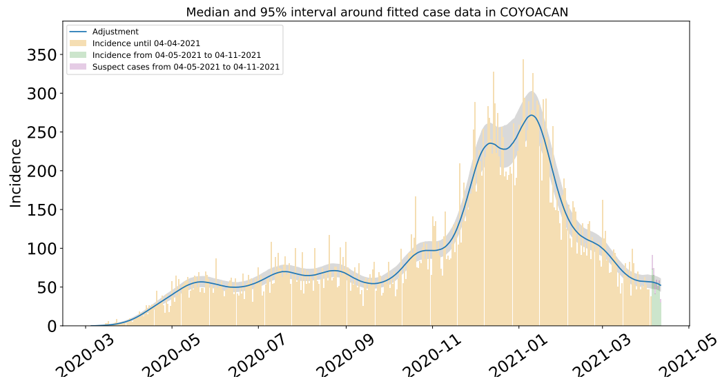
Figura 25: Ajuste de casos positivos (incidencia) por inicio de síntomas de COVID-19 en Coyoacán.
