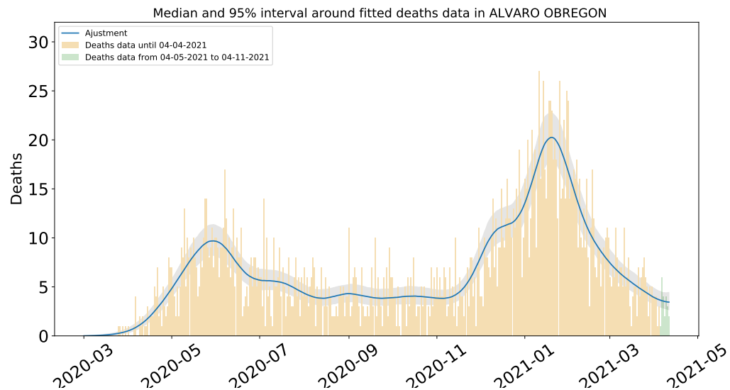
Figura 8: Ajuste y estimación de defunciones por COVID-19 para la alcaldía de Álvaro Obregón.
