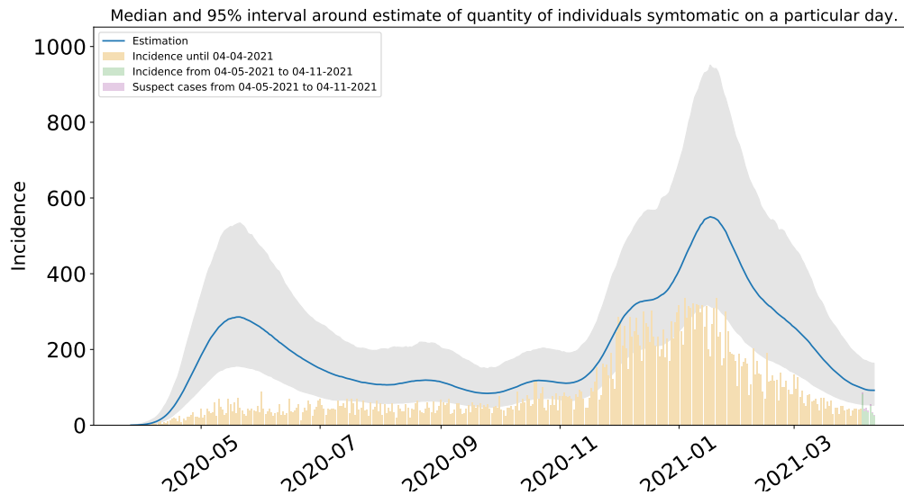
Figura 82: Estimación del número de enfermos sintomáticos en Tlaxiaco. Estimación sustentada en la proporción de infecciones sintomáticas de acuerdo a las distribuciones de covidestim (Cuadro 4 del Apéndice metodológico).
