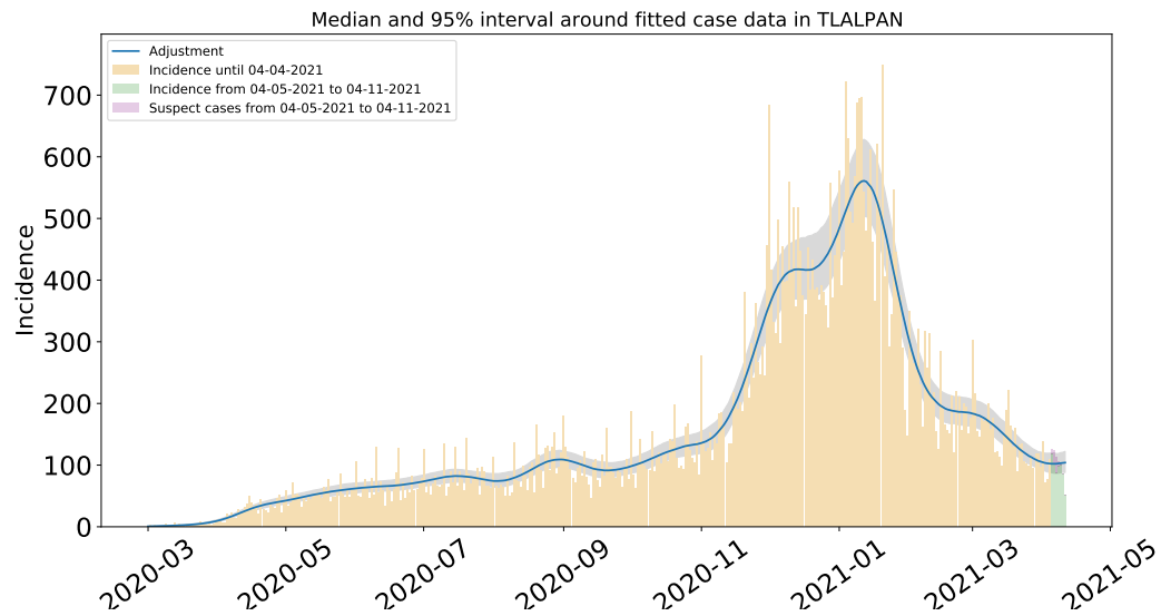
Figura 85: Ajuste de casos positivos (incidencia) por inicio de síntomas de COVID-19 en Tlalpan.
