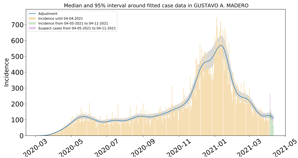
Figura 43: Ajuste de casos positivos (incidencia) por inicio de síntomas de COVID-19 en Amealco de Bonfil Gustavo A. Madero.
