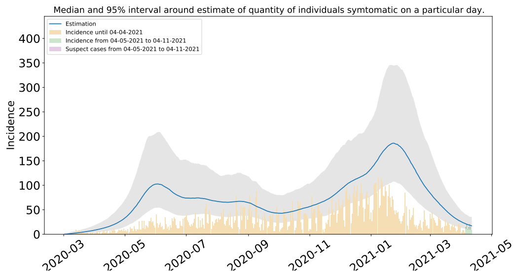
Figura 34: Estimación del número de enfermos sintomáticos en Cuajimalpa de Morelos. Estimación sustentada en la proporción de infecciones sintomáticas de acuerdo a las distribuciones de covidestim (Cuadro 4 del Apéndice metodológico).
