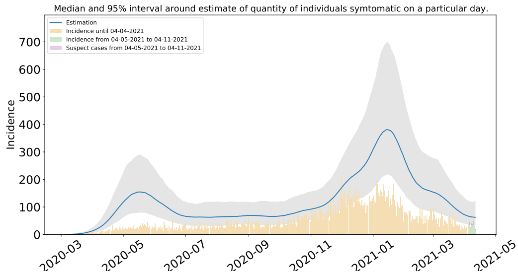
Figura 22: Estimación del número de enfermos sintomáticos en Benito Juárez. Estimación sustentada en la proporción de infecciones sintomáticas de acuerdo a las distribuciones de covidestim (Cuadro 4 del Apéndice metodológico).
