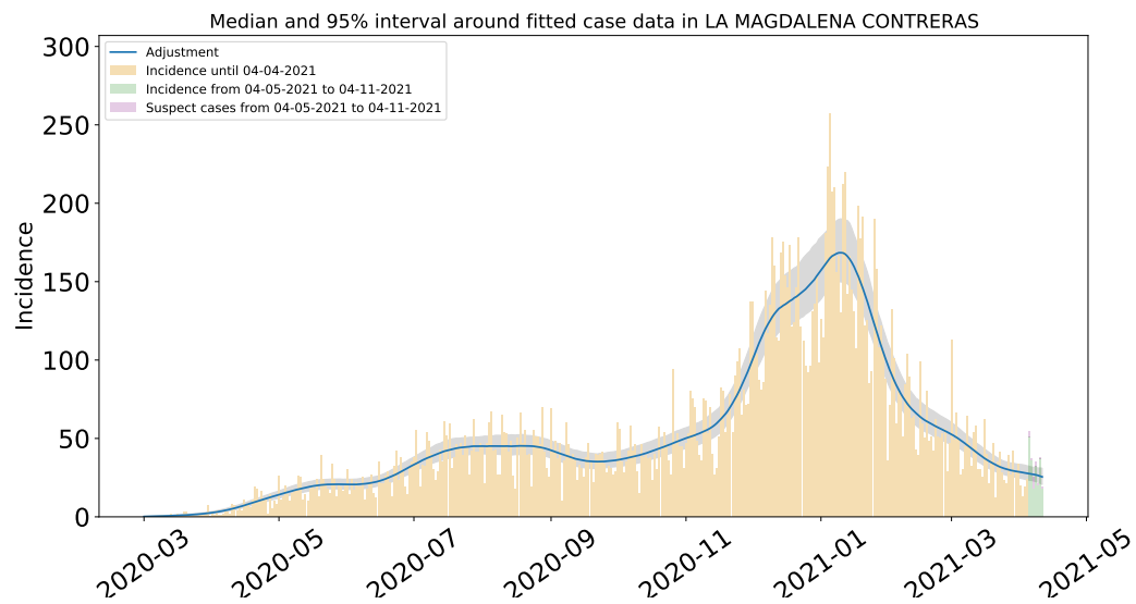
Figura 61: Ajuste de casos positivos (incidencia) por inicio de síntomas de COVID-19 en Magdalena Contreras.
