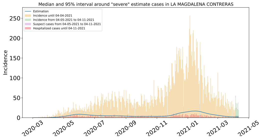
Figura 63: Estimación de casos severos de COVID-19 en la alcaldía Magdalena Contreras comparada con los casos hospitalizados reportados.
