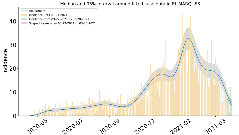
Figura 37: Ajuste y estimación de casos positivos de COVID-19 por inicio de síntomas en El Marqués usando la paquetería covidestim con las densidades a priori nacionales y datos actualizados el 11 de abril de 2021, recortados hasta el 4 de abril de 2021.
